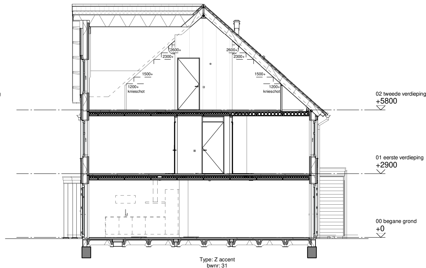
Doorsnede B
