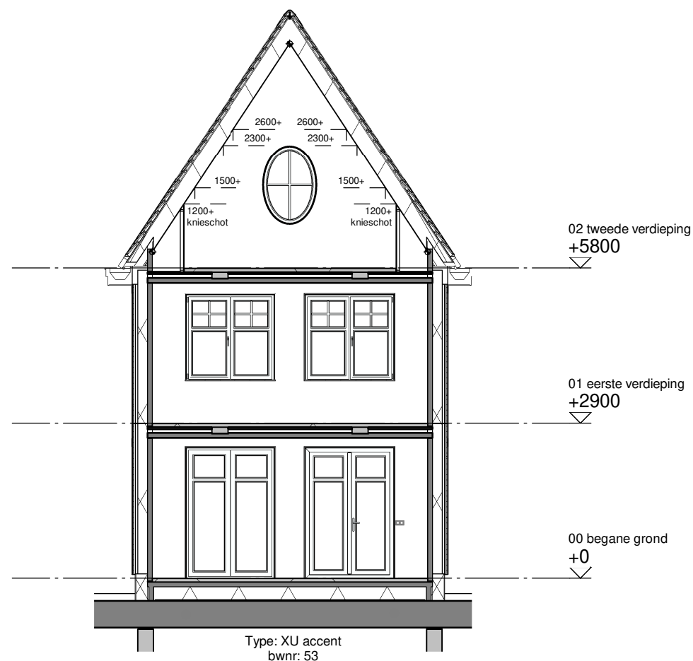
Doorsnede C
