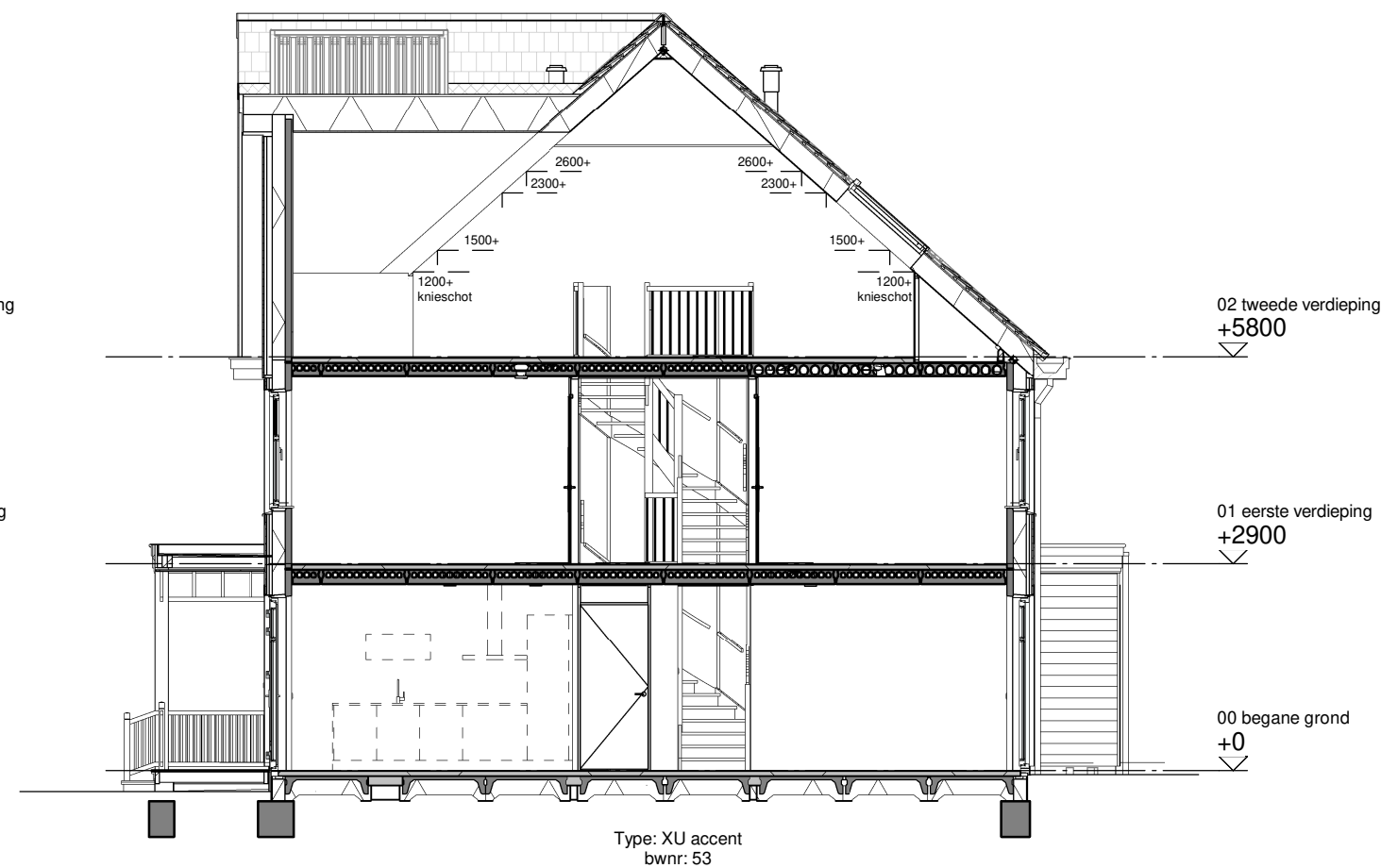
Doorsnede B
