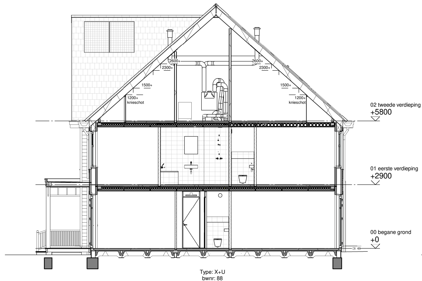
Doorsnede A
