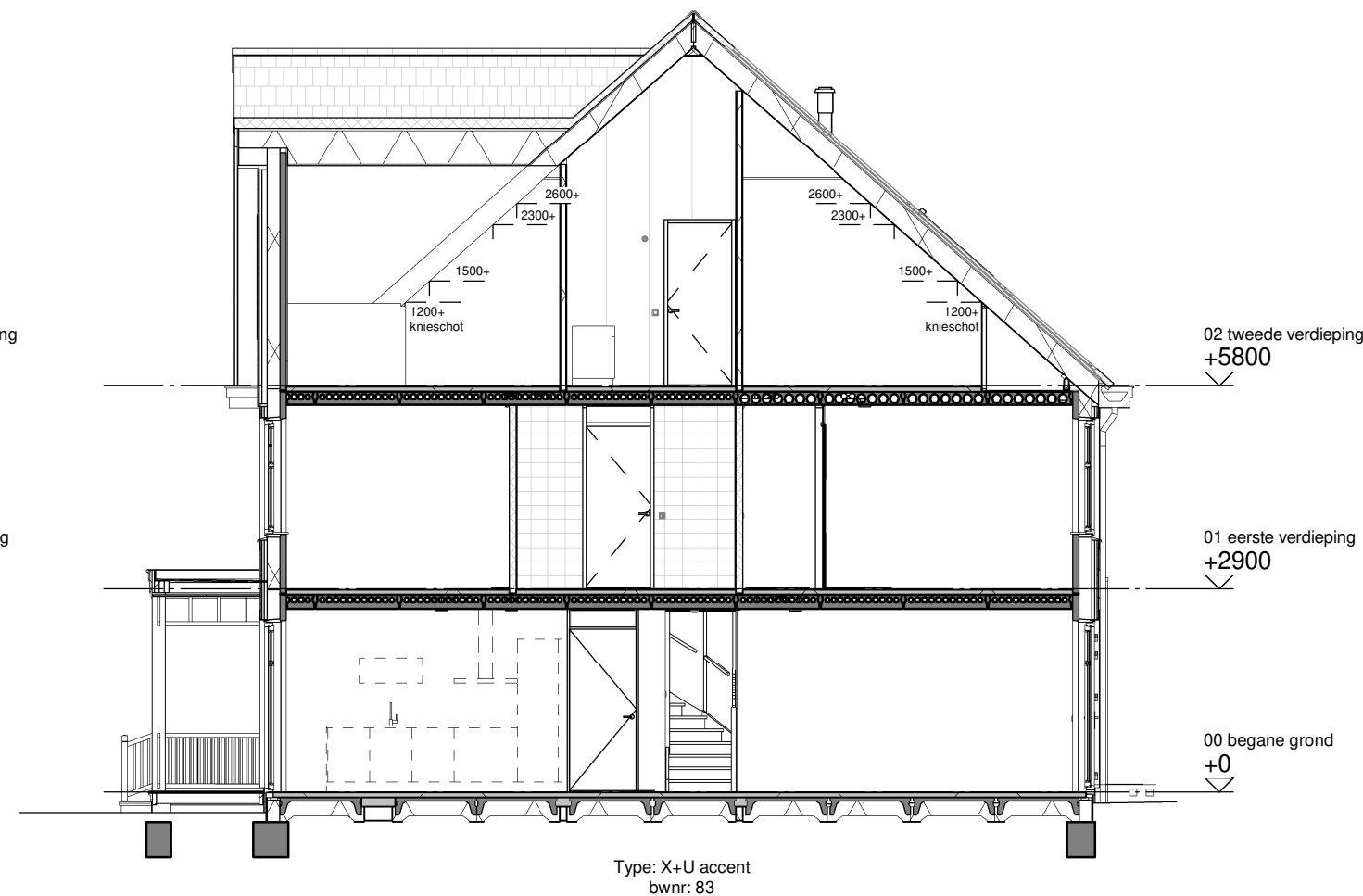
Doorsnede B
