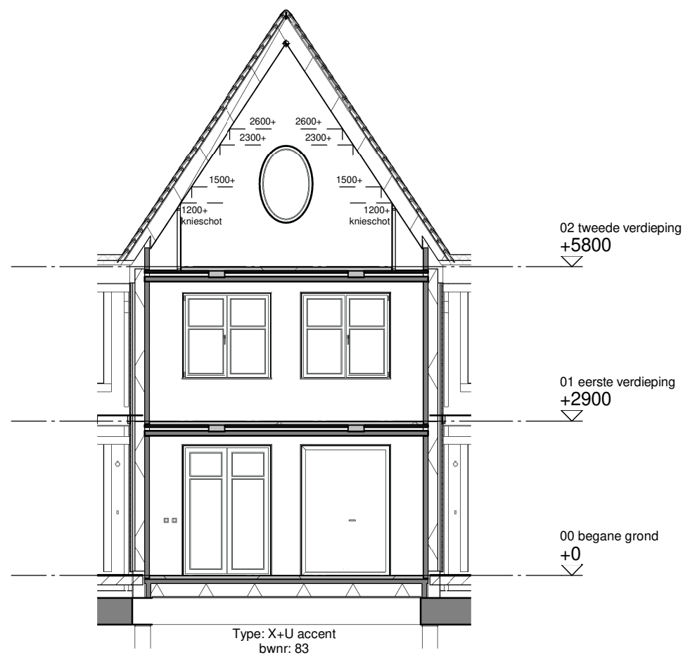
Doorsnede C
