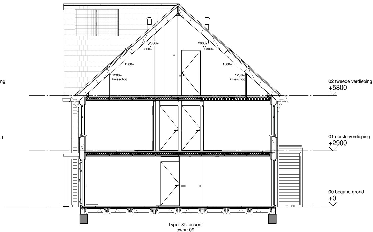
Doorsnede B
