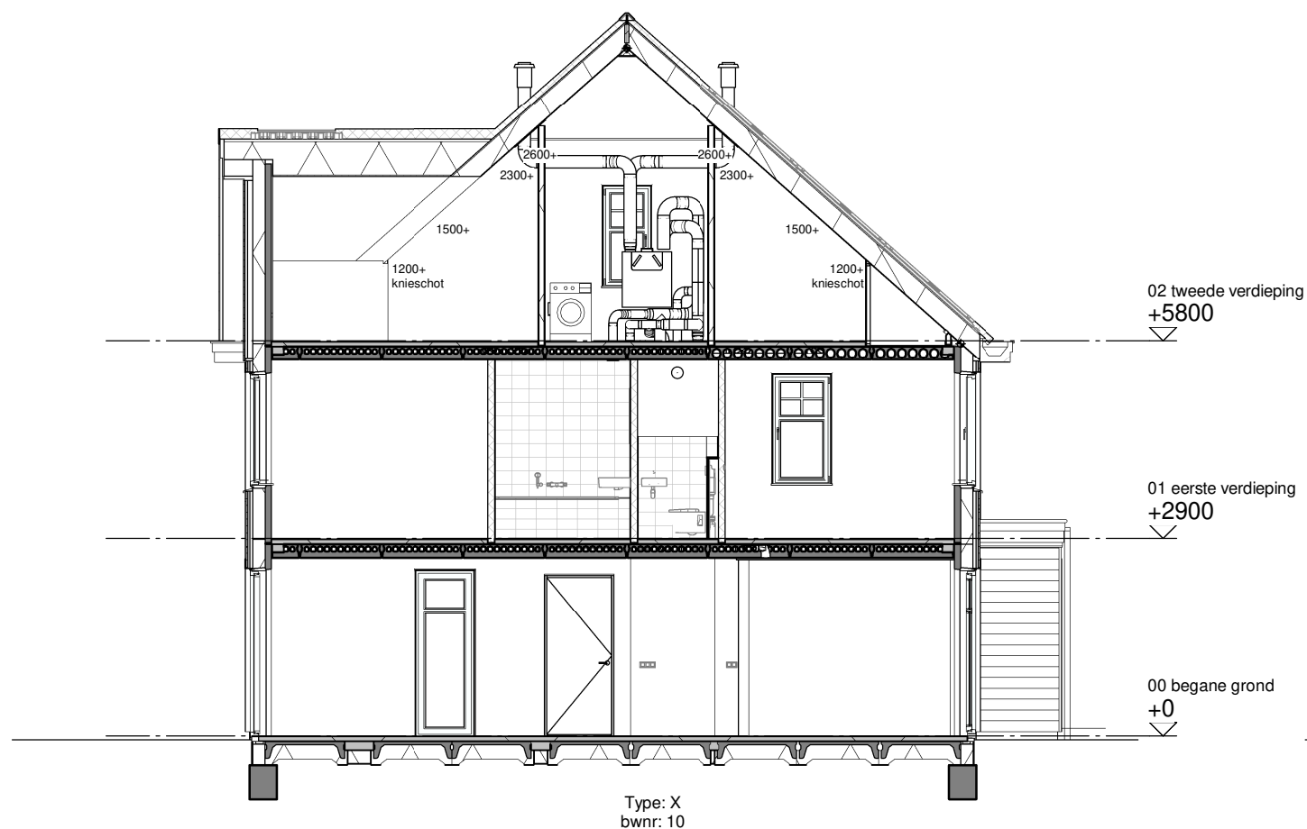
Doorsnede A
