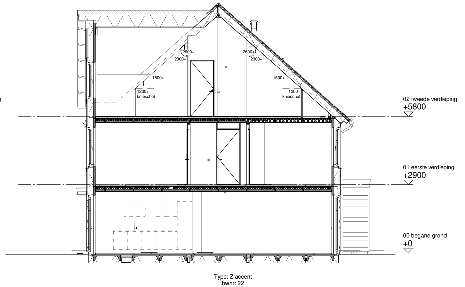
Doorsnede B
