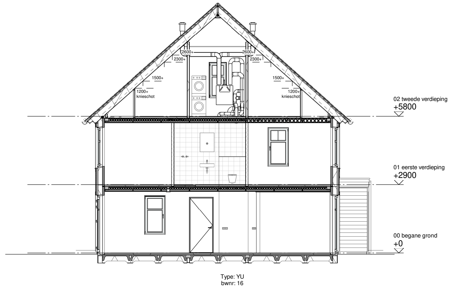
Doorsnede A
