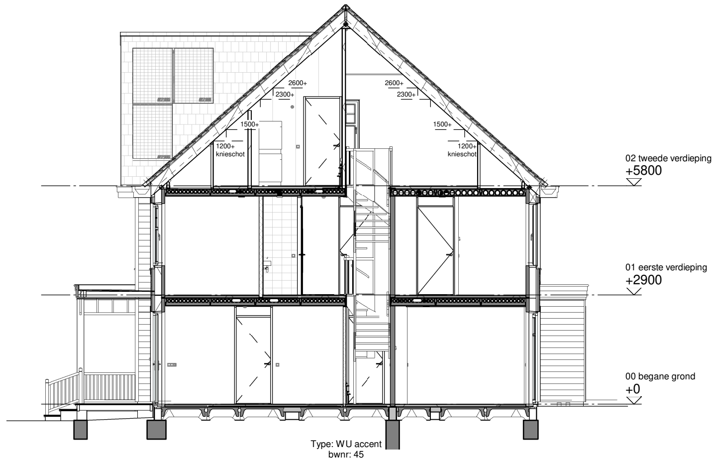
Doorsnede A
