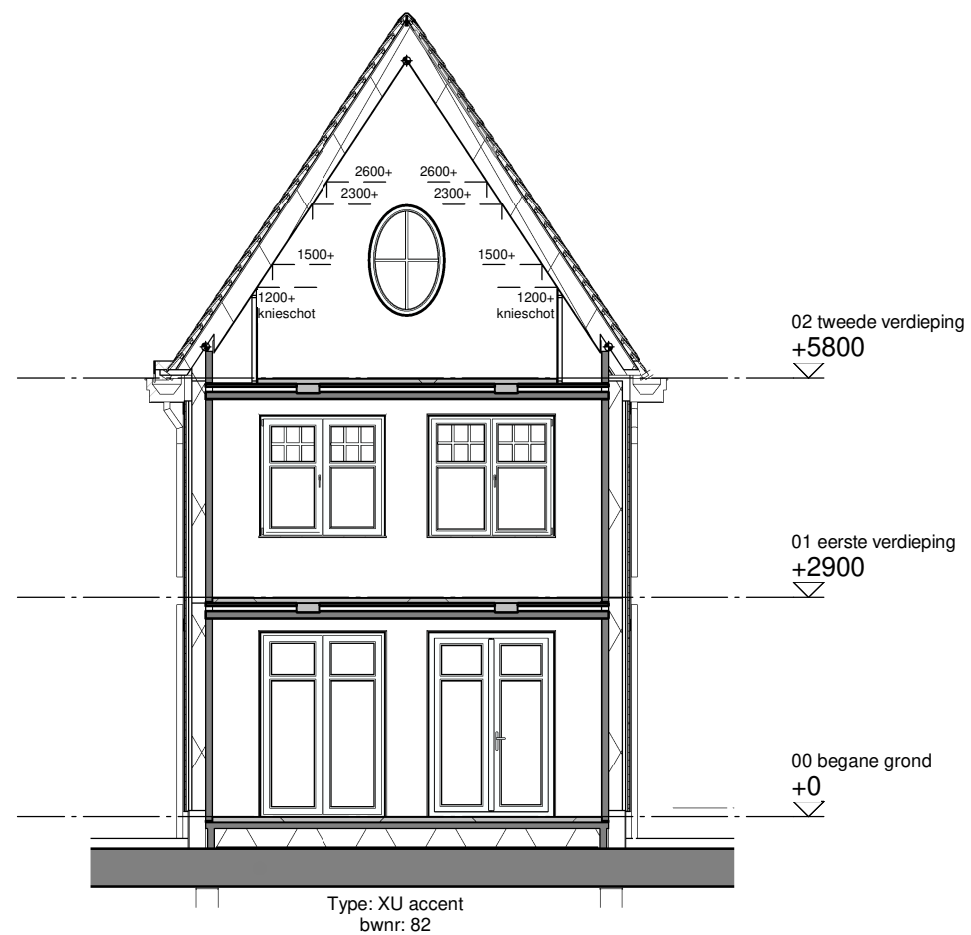
Doorsnede C
