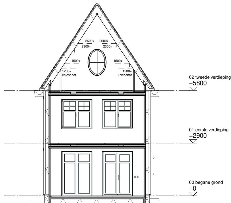
Doorsnede A
