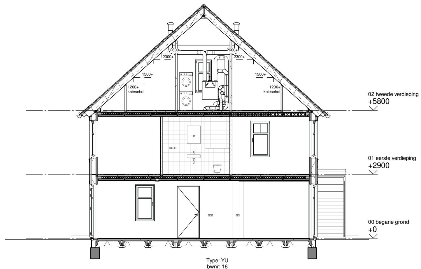
Doorsnede A
