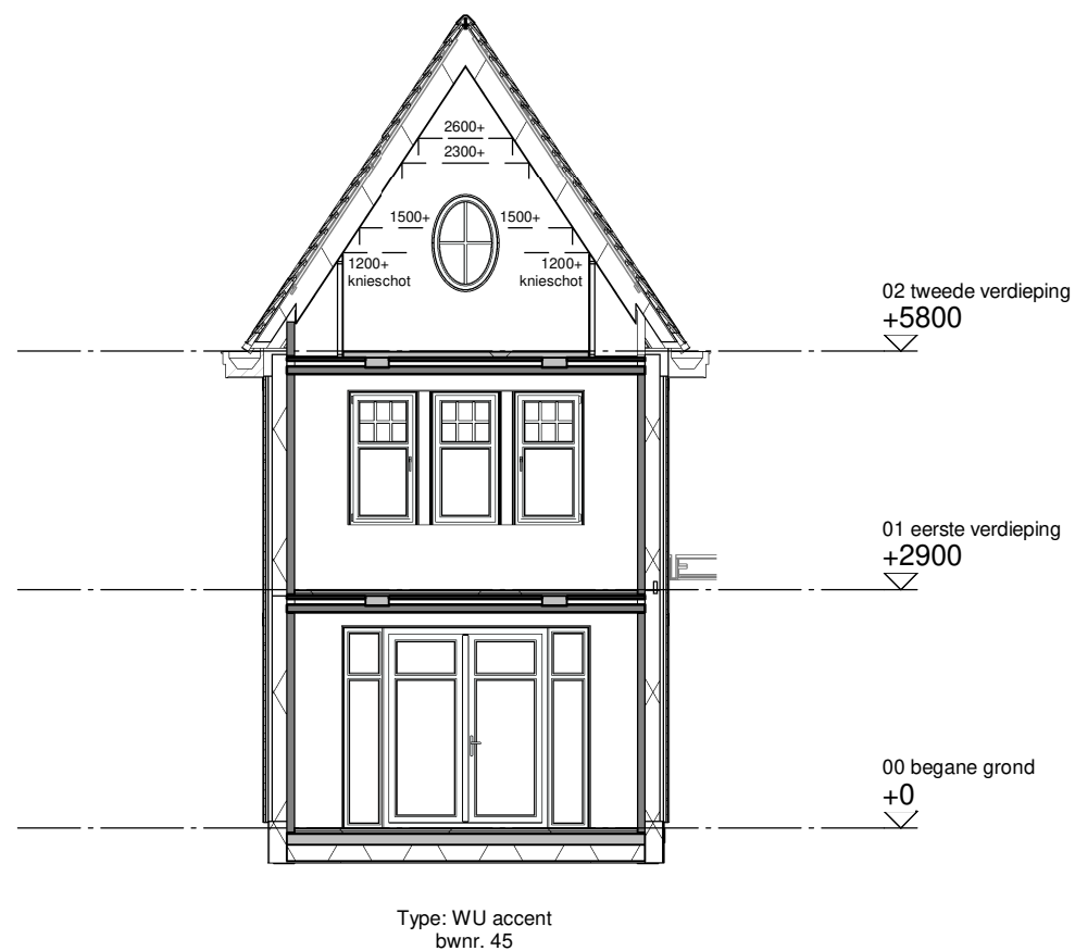
Doorsnede C
