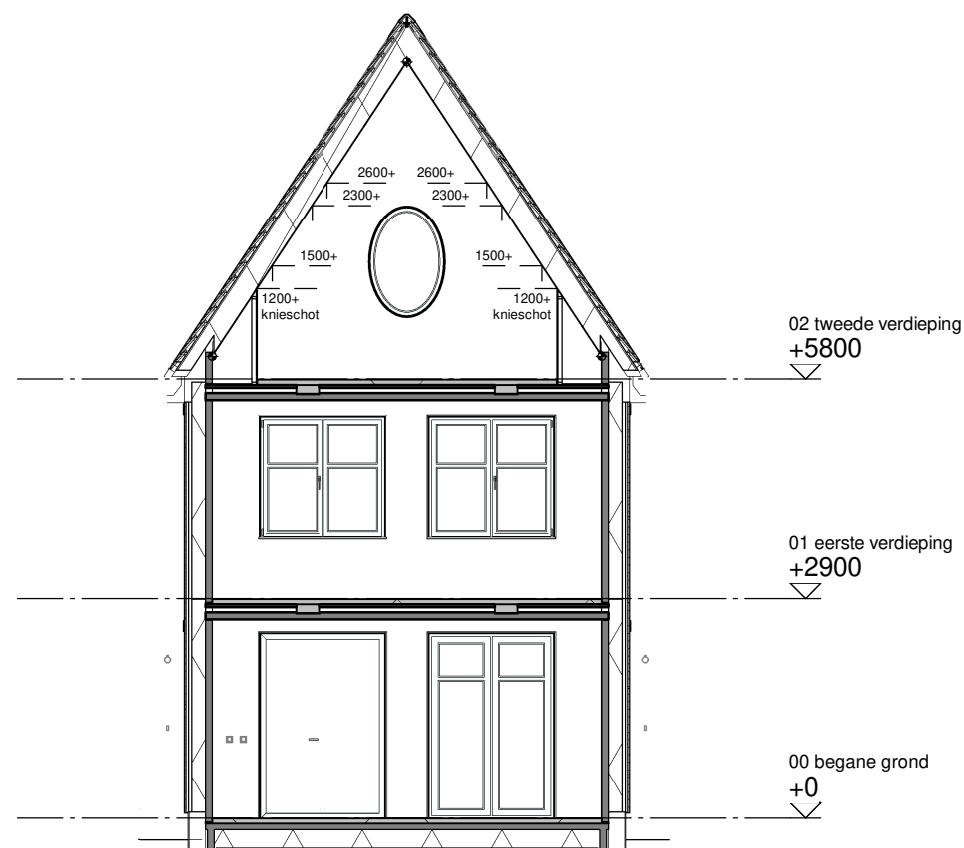
Doorsnede A
