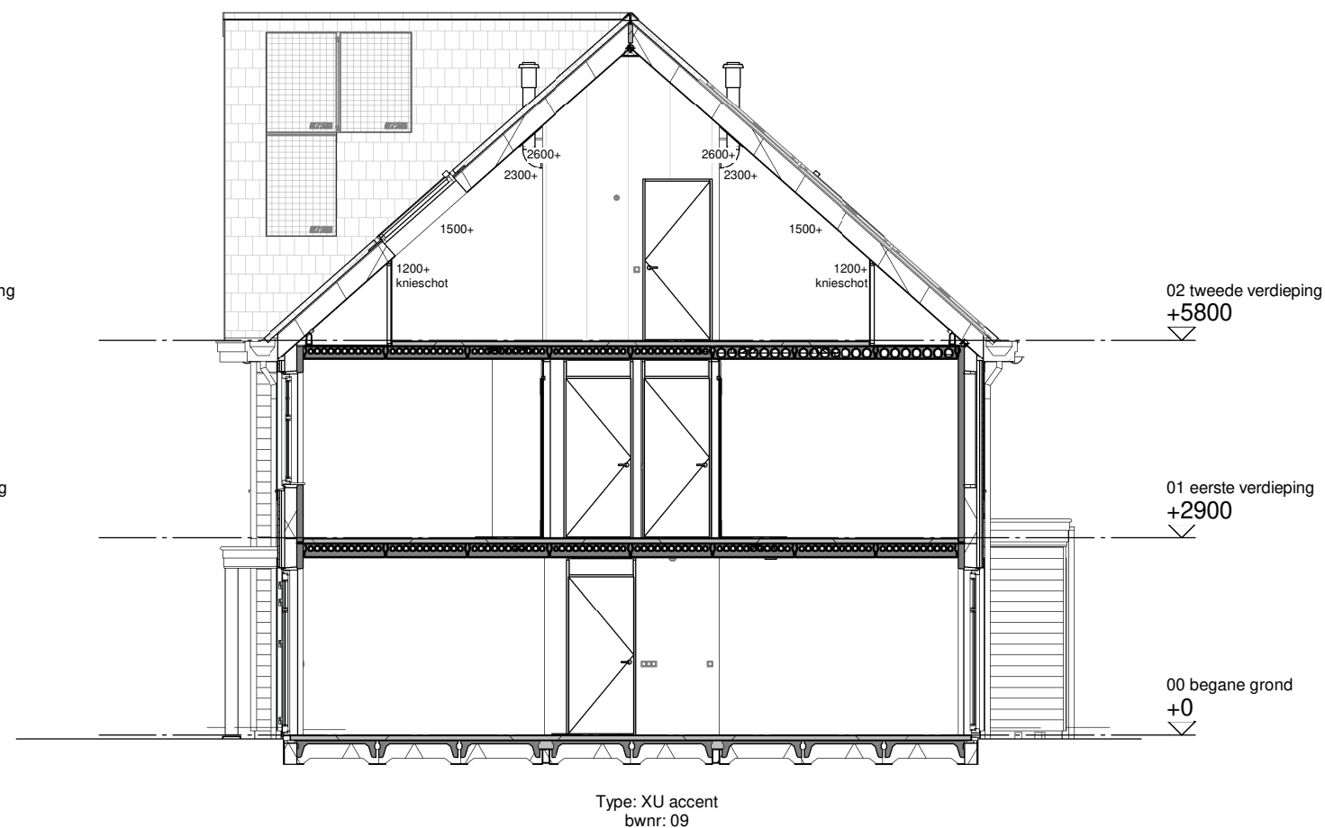
Doorsnede B
