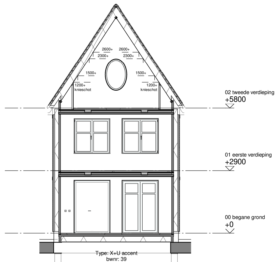
Doorsnede C
