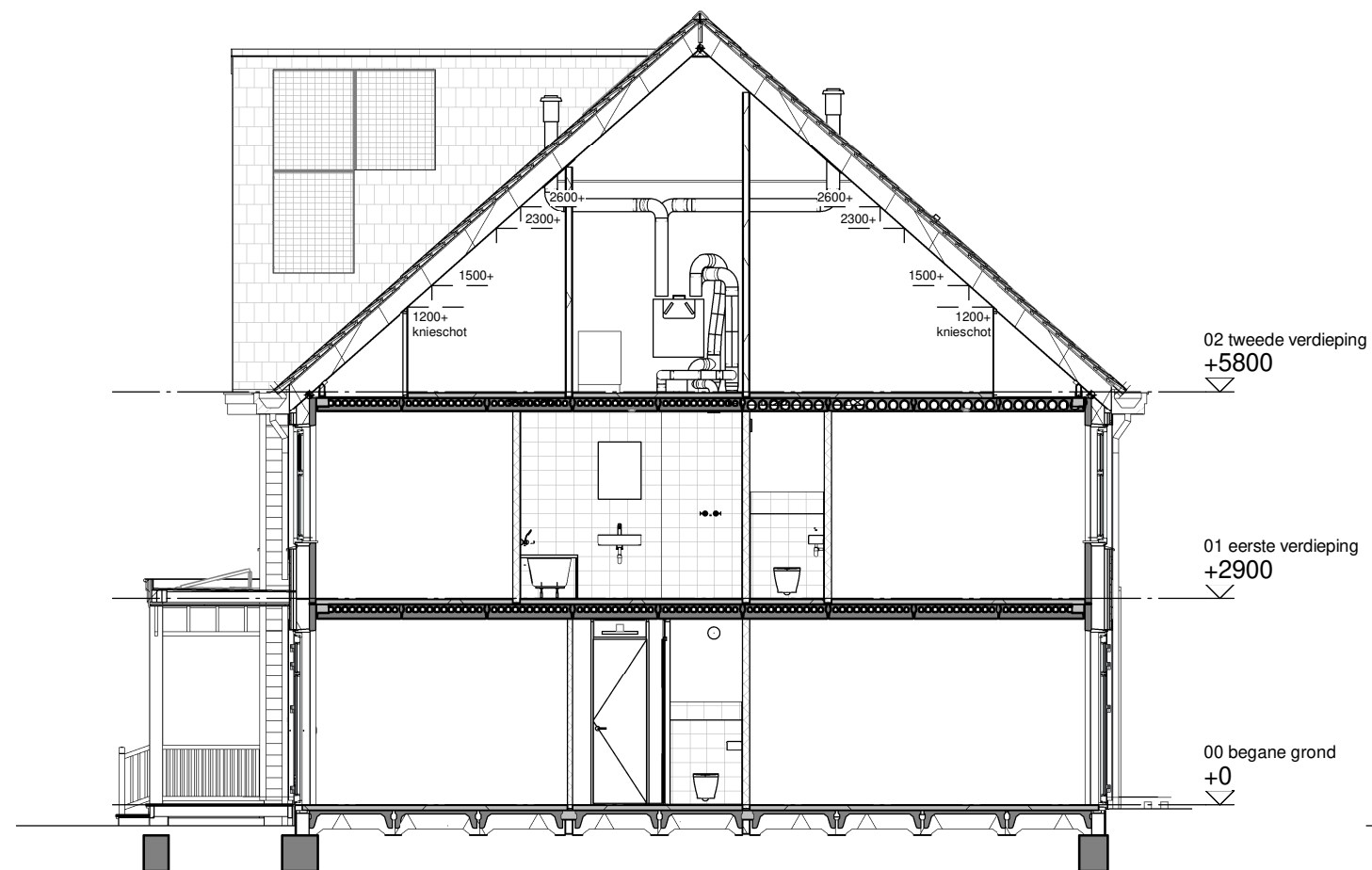
Doorsnede A
